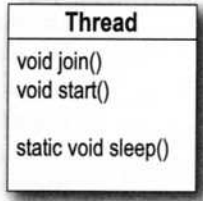
java.lang.Thread class
